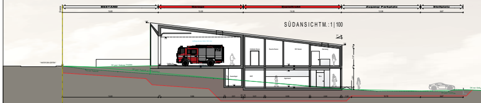
ENTWURF FEUERWEHRGERÄTEHAUS ROHRBACH VERSION 03/10.01.2018
