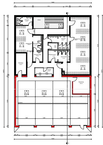
ENTWURF FEUERWEHRGERÄTEHAUS ROHRBACH VERSION 03/10.01.2018
